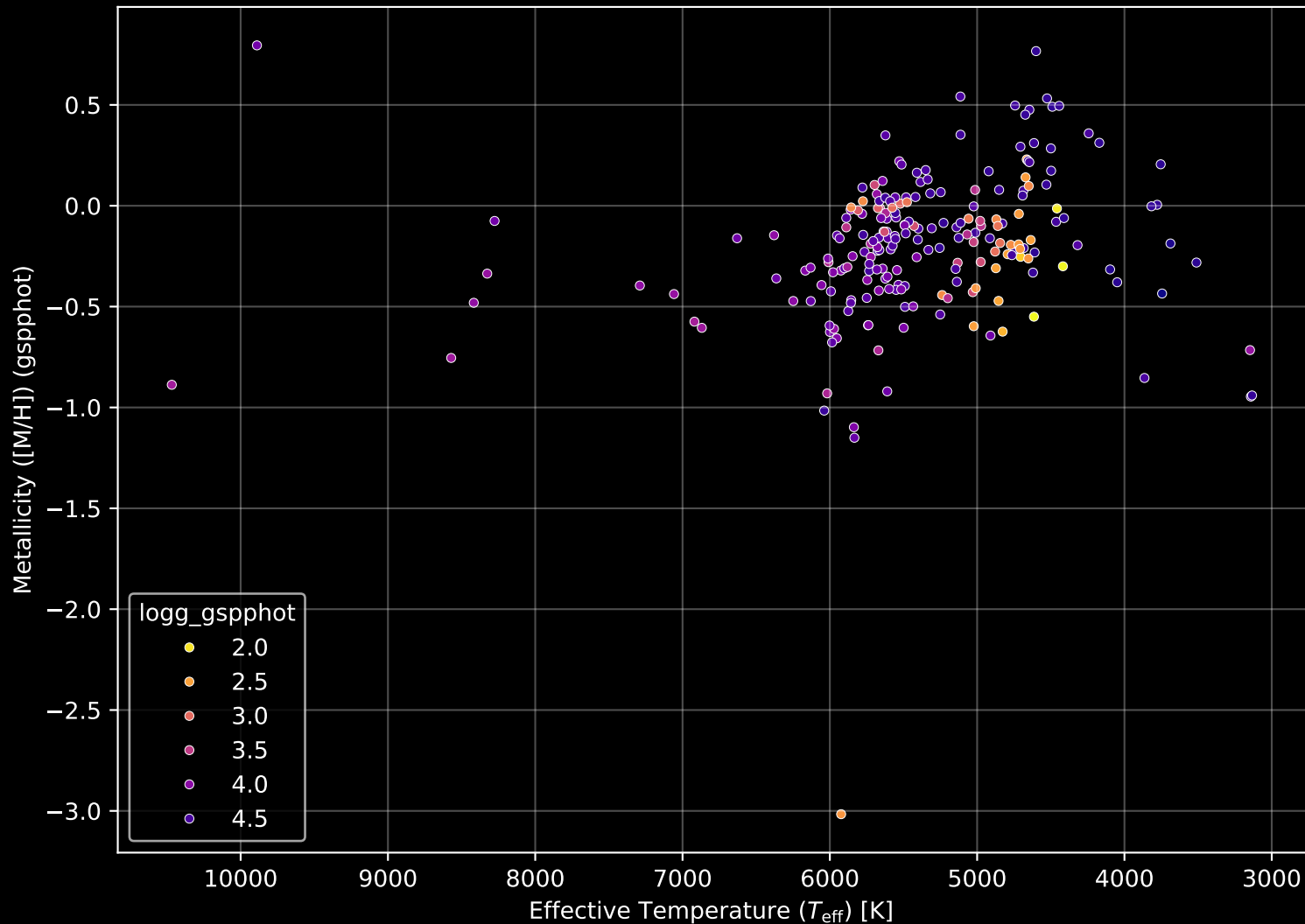
APOGEE DR17 Field: [235+42_MGA] Stellar Population Parameters (n= 216)
